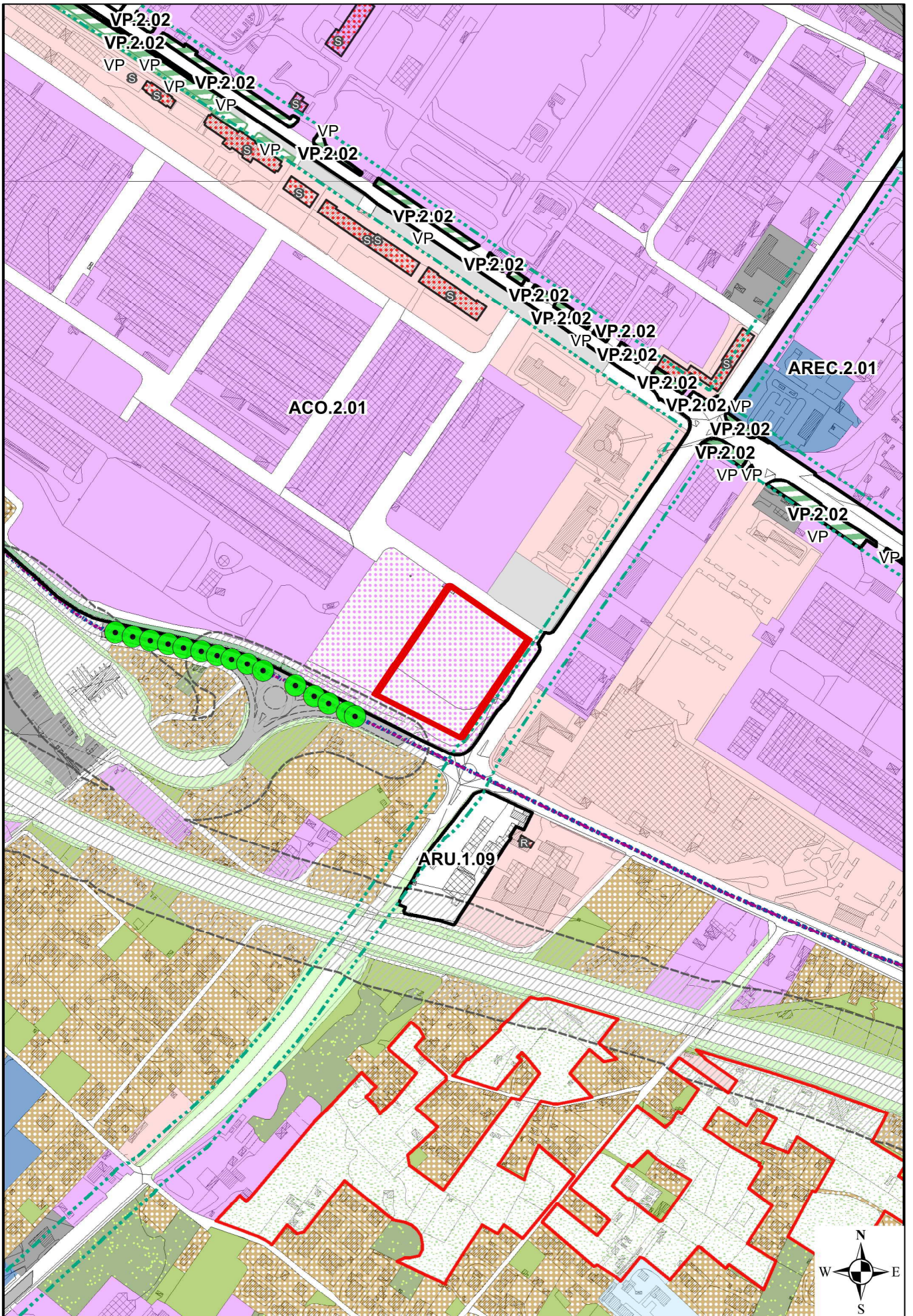
STRALCIO TAVOLA QP1 - SCALA 1:5000
