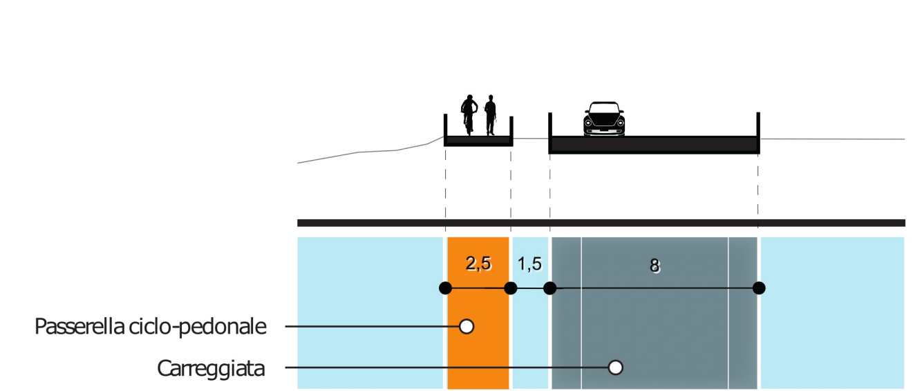
SEZIONE DD'
