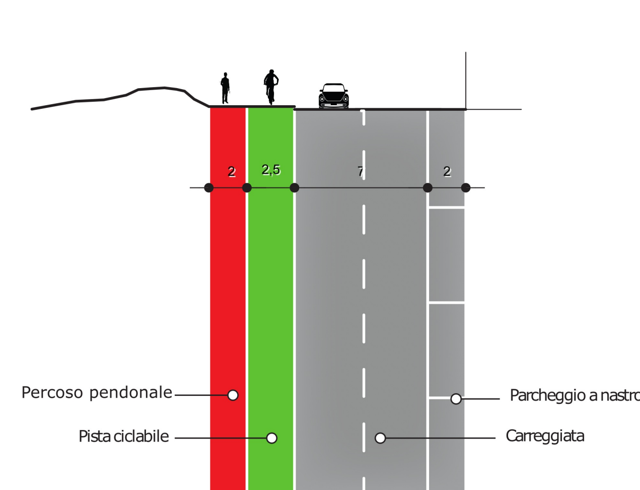
SEZIONE FF'
