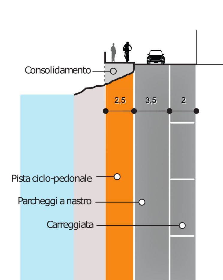
SEZIONE CC'
