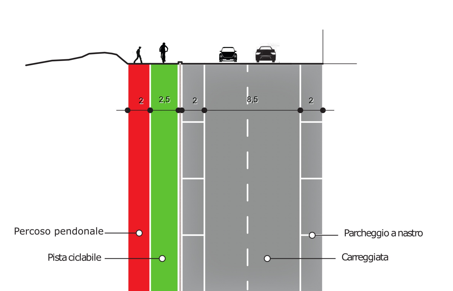
SEZIONE GG'
