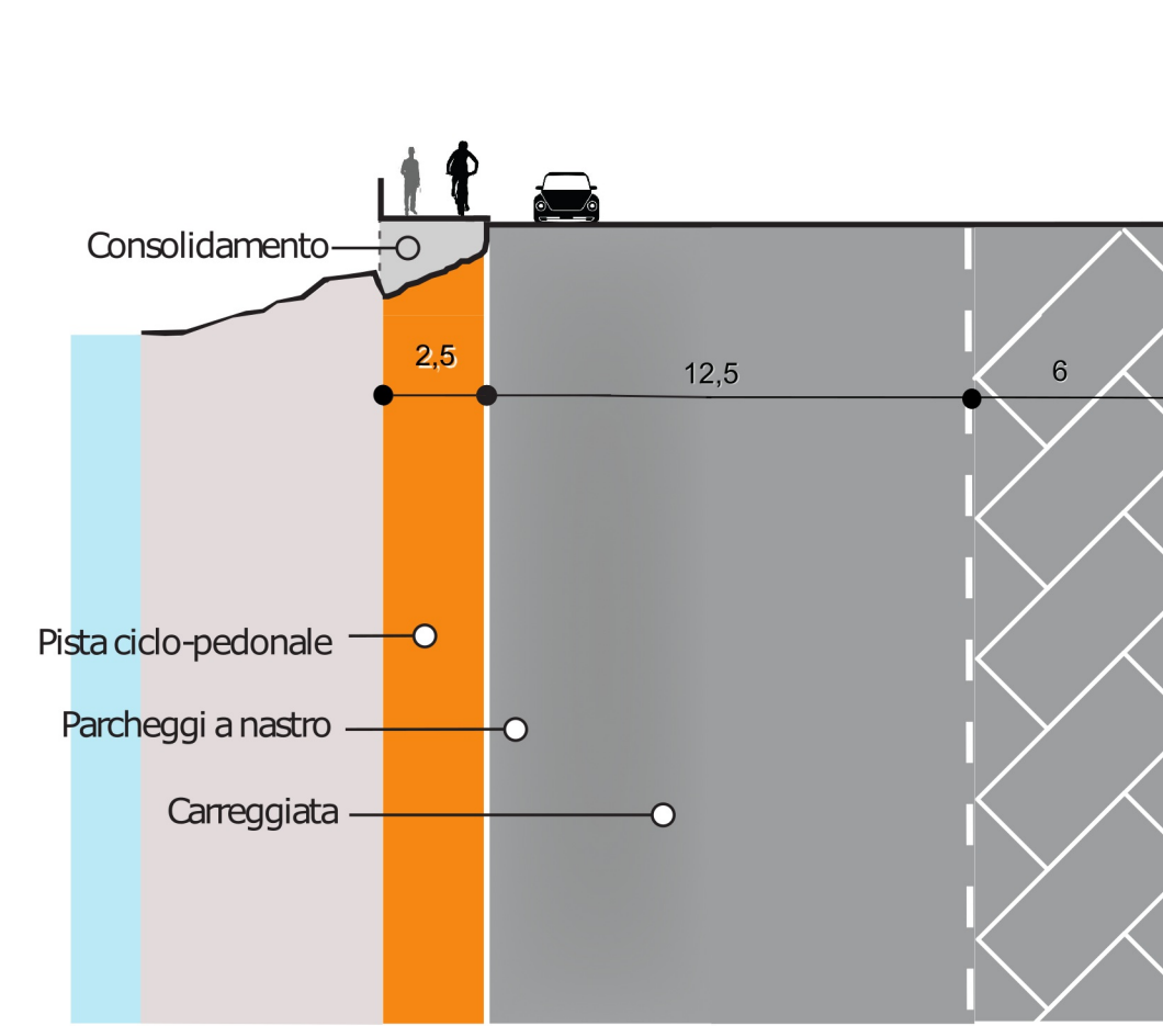
SEZIONE BB'
