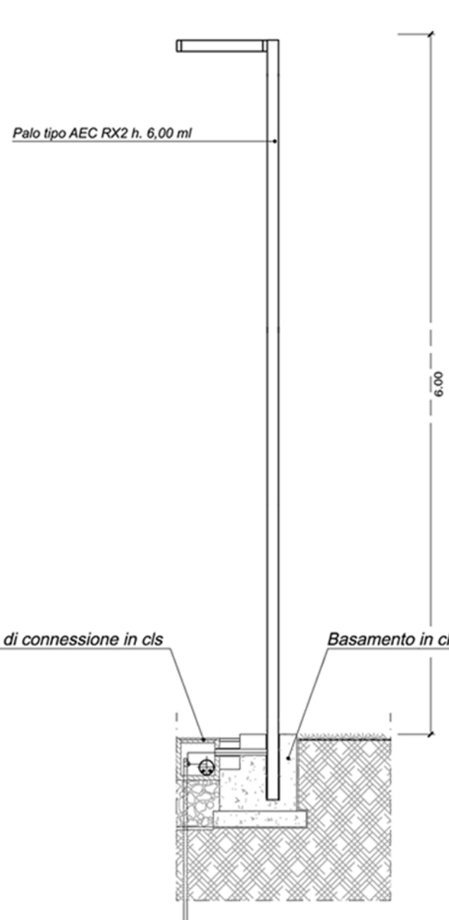
Particolare fondazione e pozzetto palo AEC RX2
