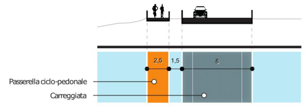
SEZIONE DD'
