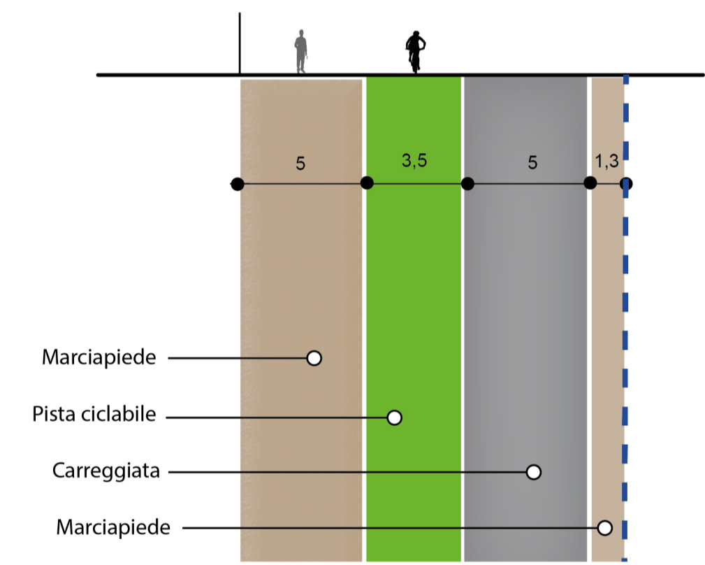
SEZIONE AA'
