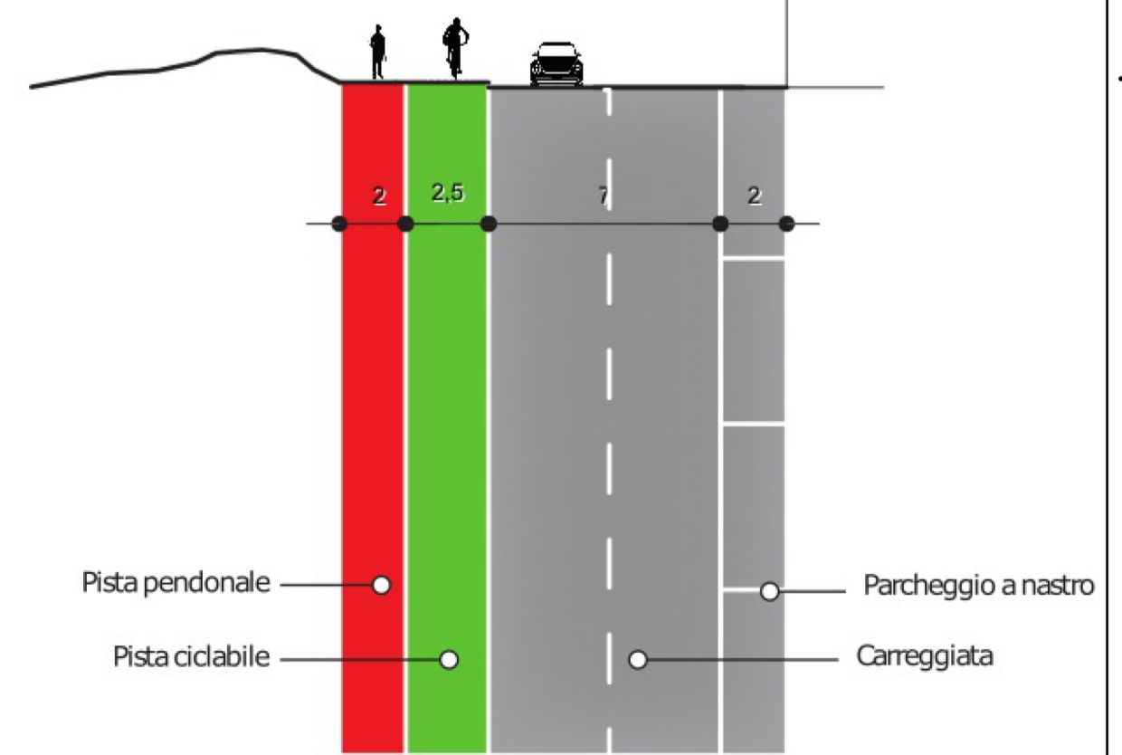
SEZIONE FF'
