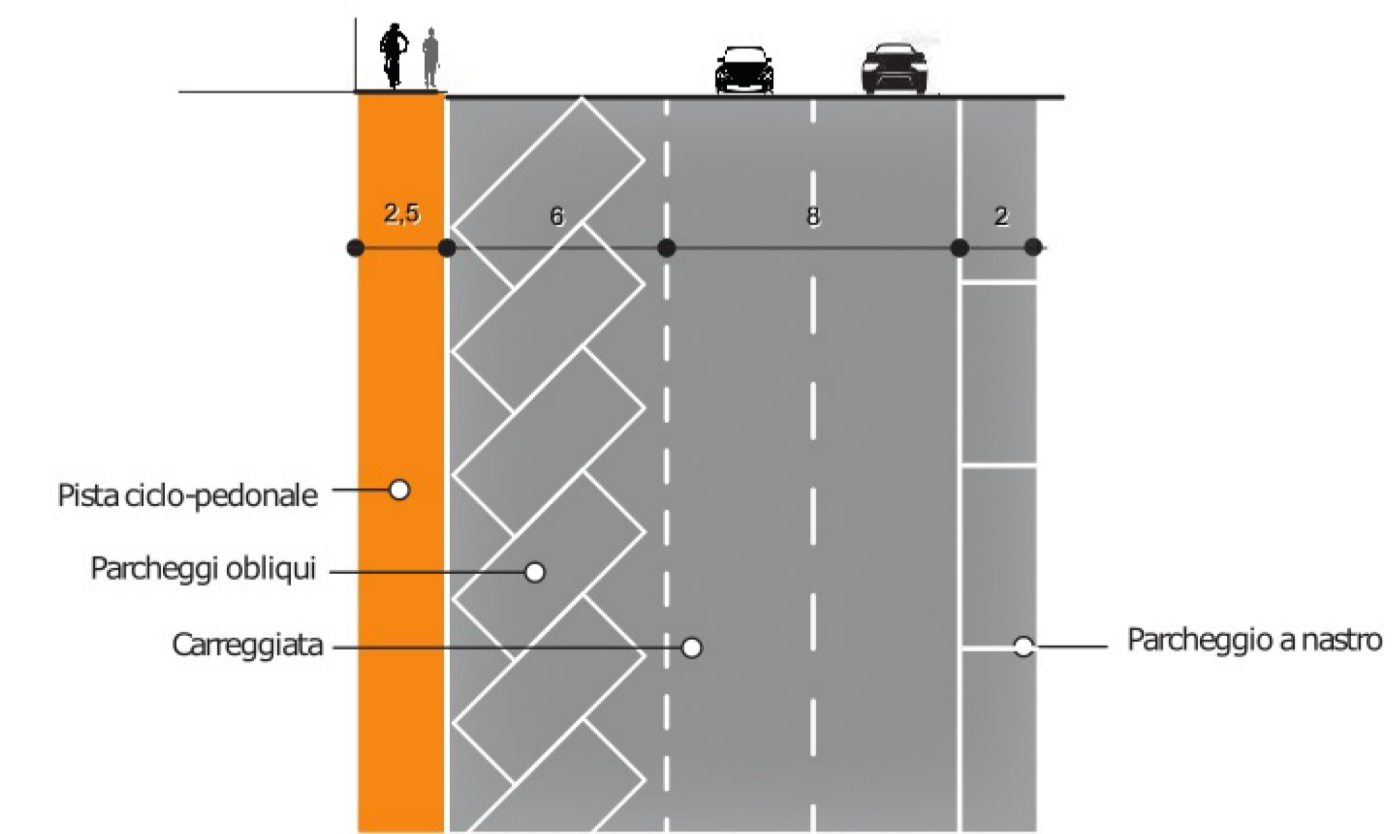
SEZIONE EE'
