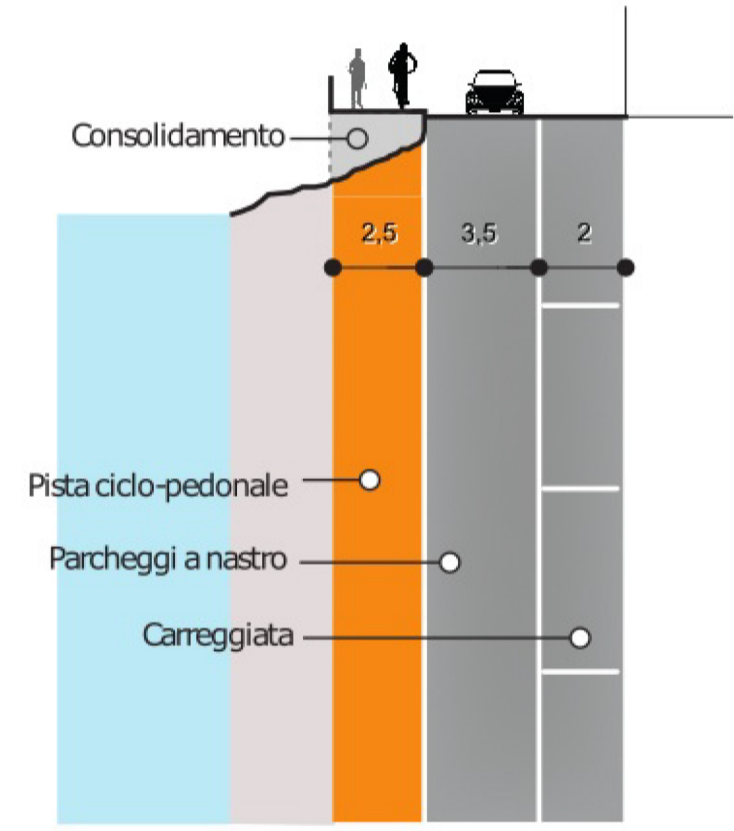
SEZIONE CC'
