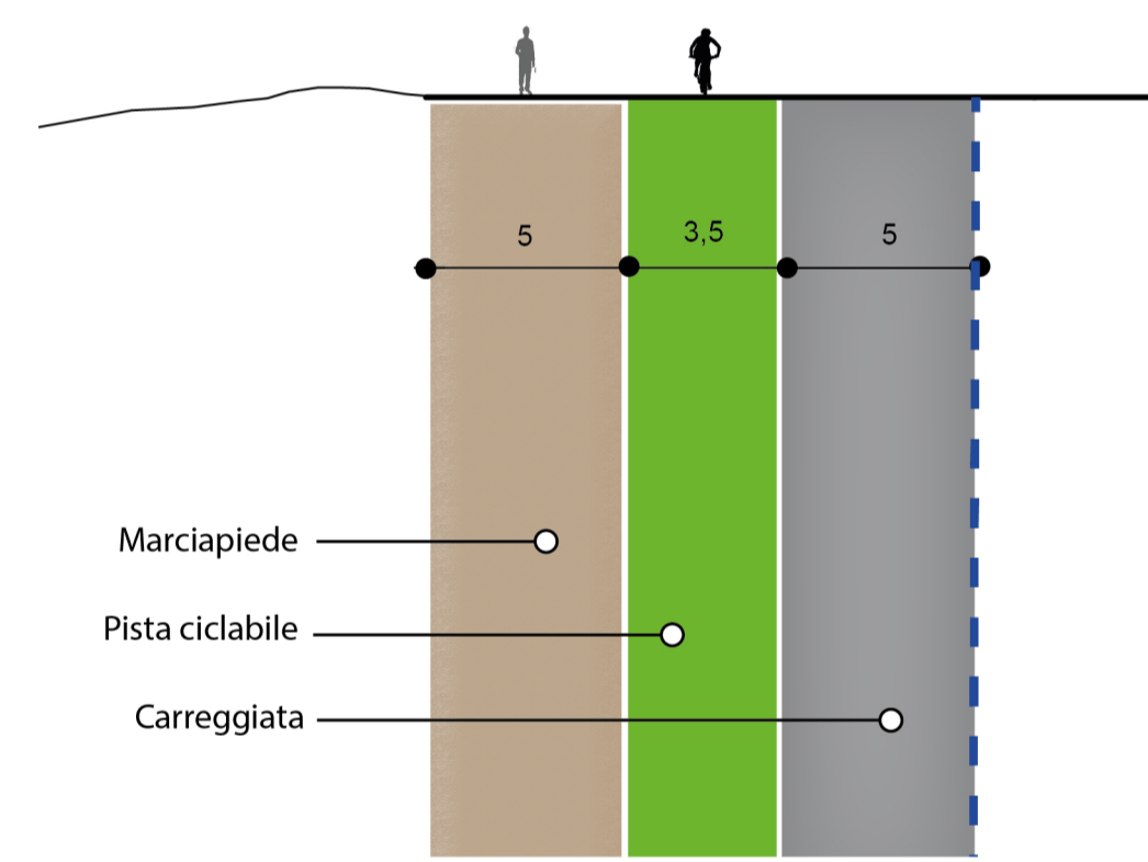
SEZIONE BB'
