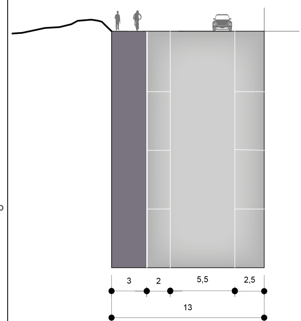
SEZIONE GG'
