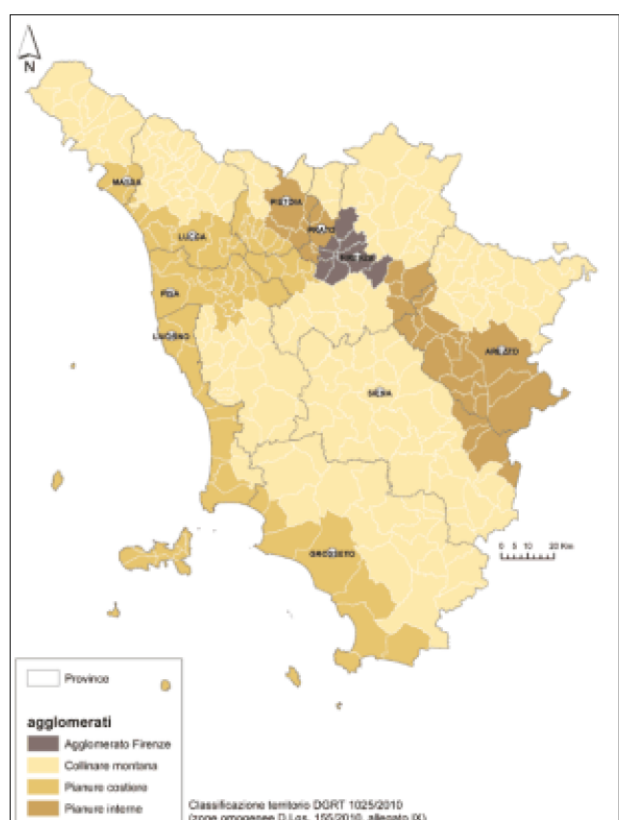
Figura 4.6 - Suddivisione del territorio regionale per l'ozono
