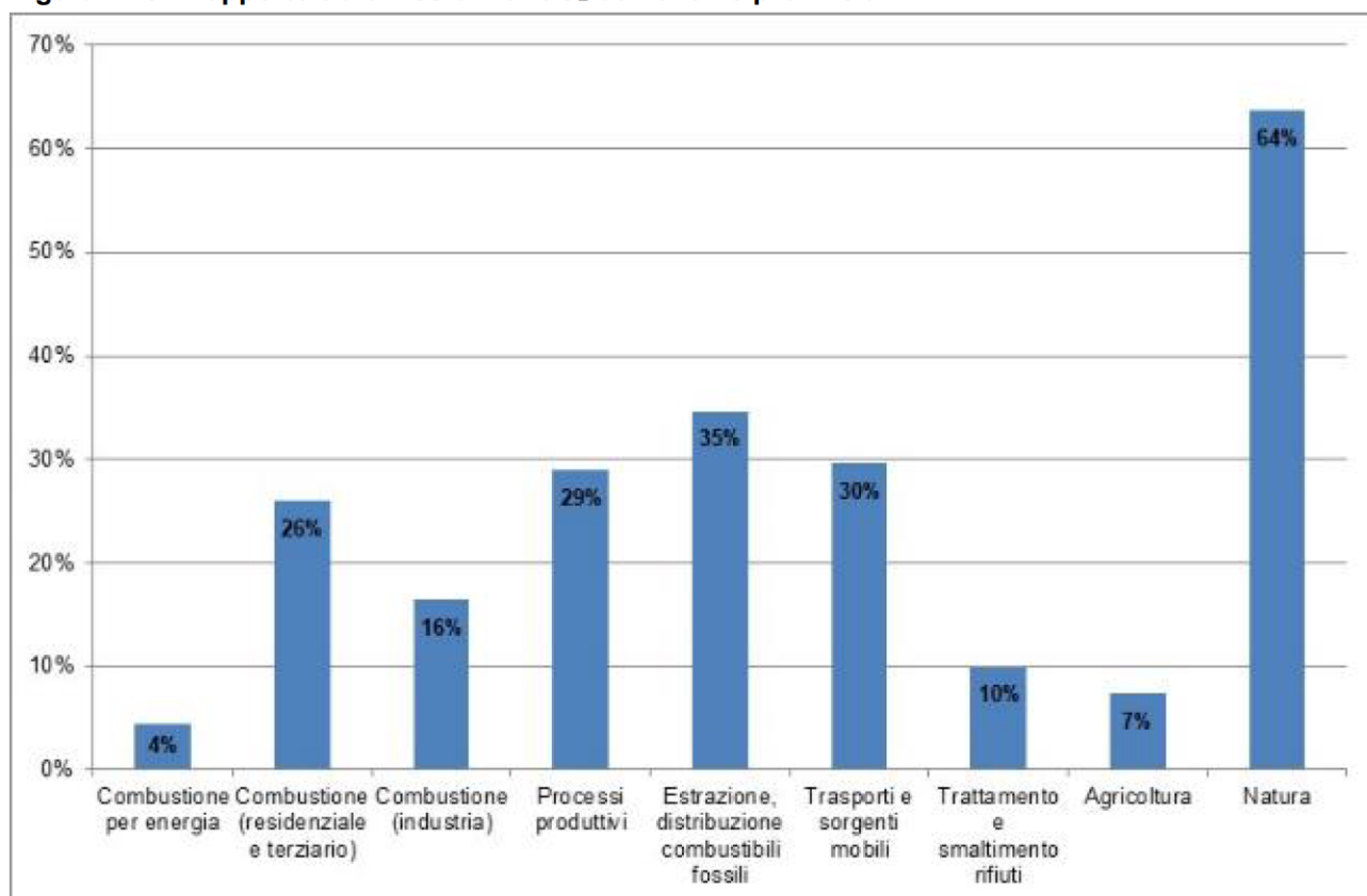
Figura 4.23 - Rapporto tra emissioni di CO 2 comunali e provinciali
