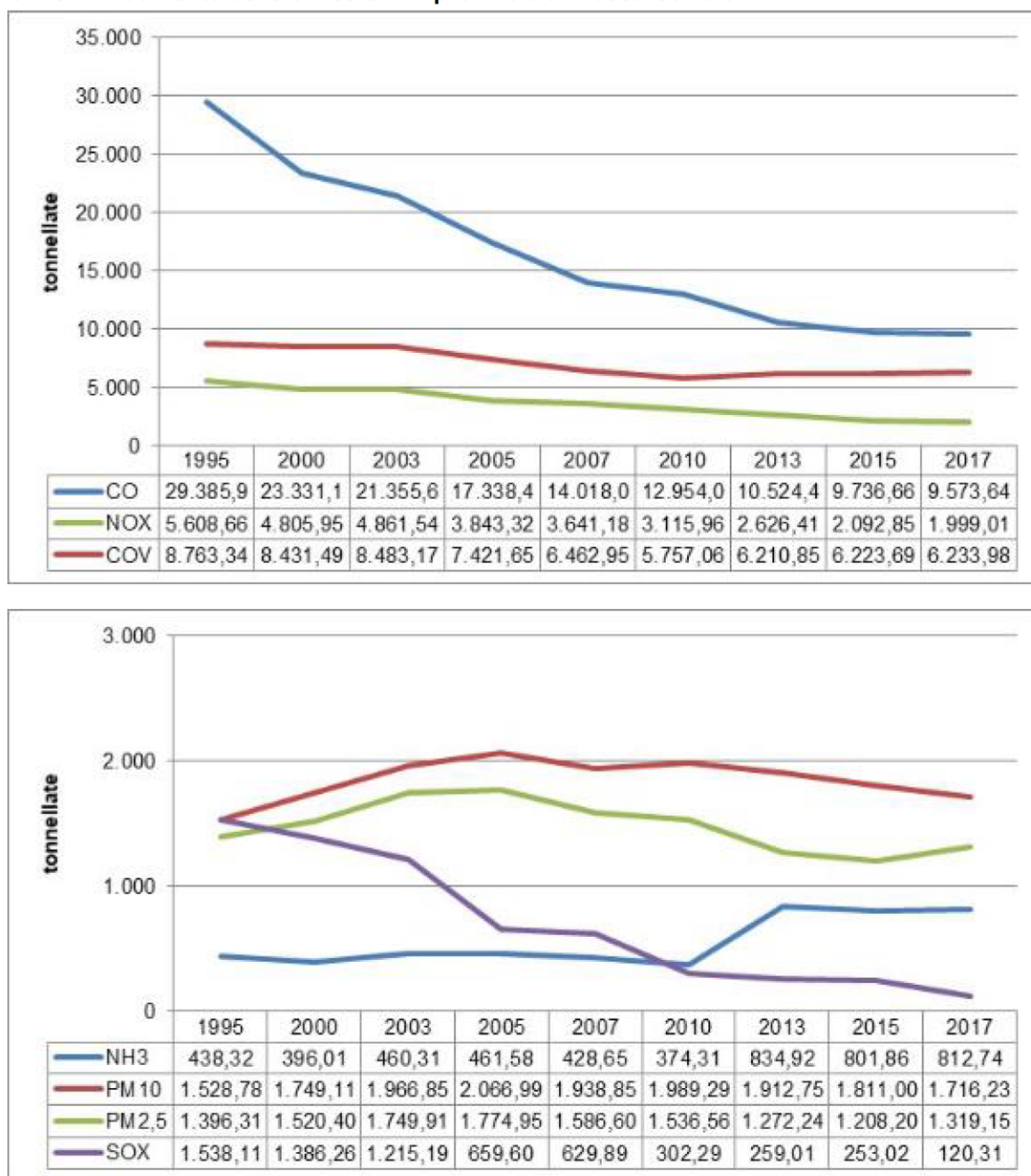
Figura 4.8 – Andamento delle emissioni in provincia di Massa-Carrara
