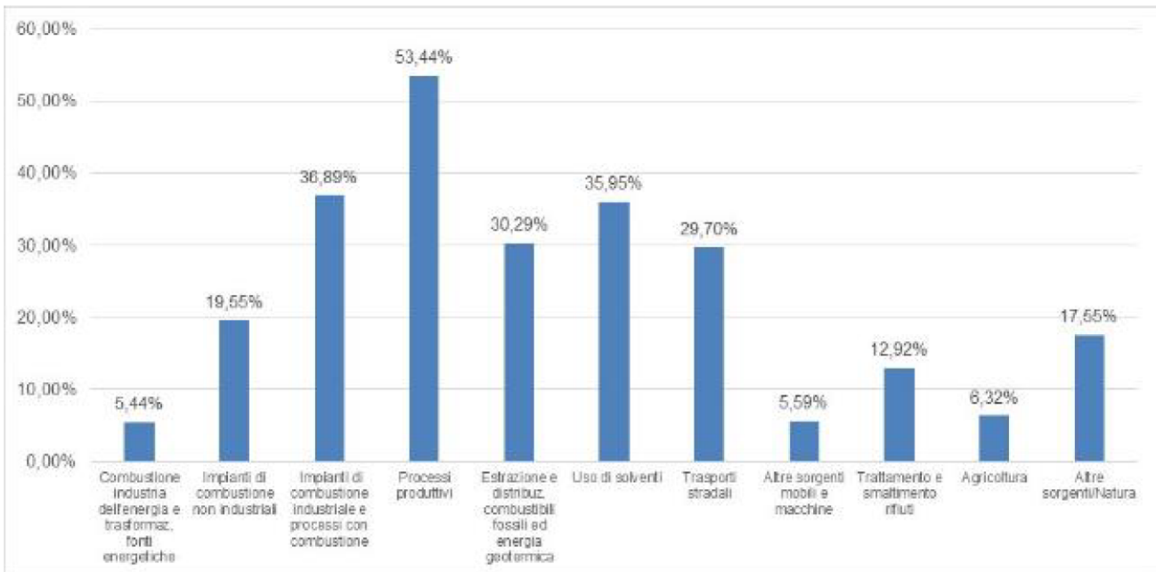
Figura 4.11 - Contributo del comune di Massa alle emissioni provinciali suddivise per macrosettori: anno 2017
